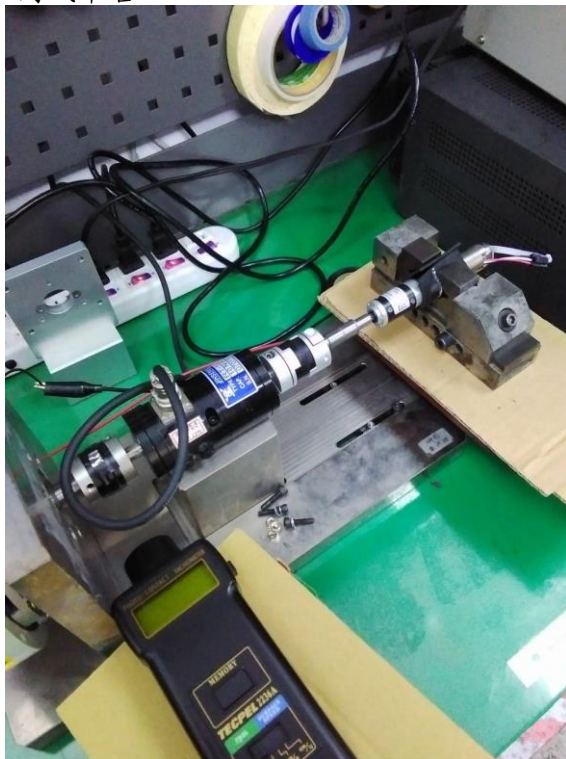
測試平台
