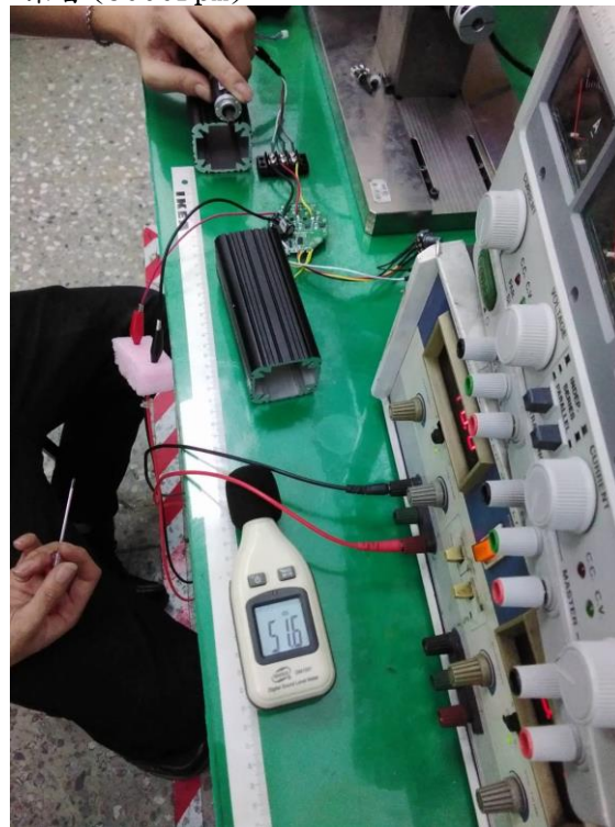
噪音(5000rpm)
